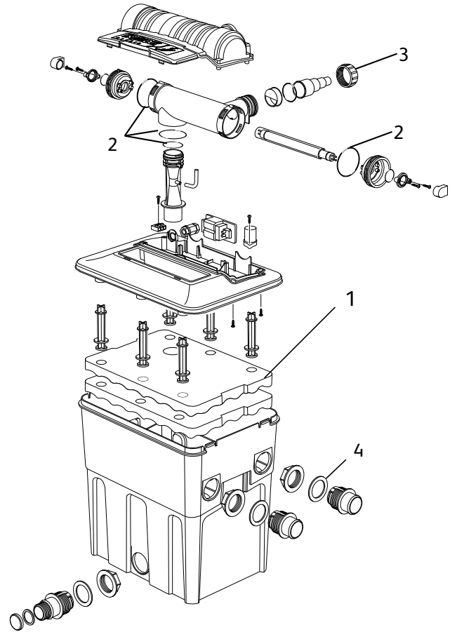
Ecomax 4500 & 9000 Ecopower+ 5000/10000 & 10000/20000
